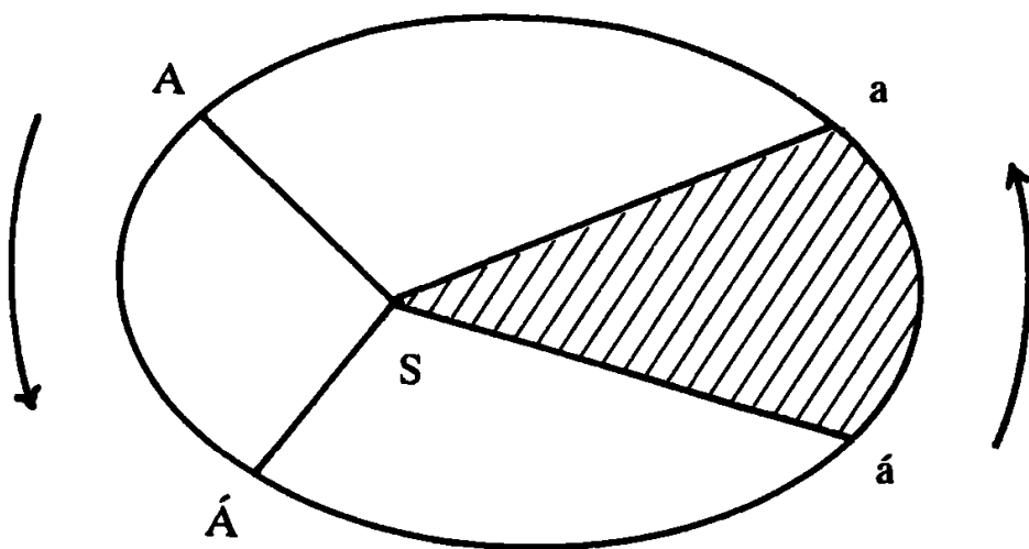
تصویری از مدار بیضی گونه کپلر
