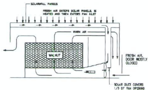
شکل ۱۳ - خشک کن خورشیدی
