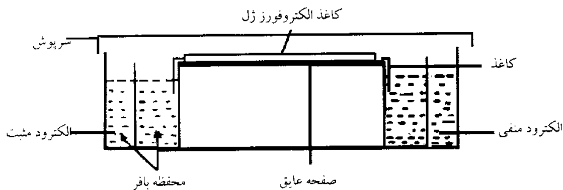
شکل ۱۴-۳ دستگاه الکتروفورز کاغذی
