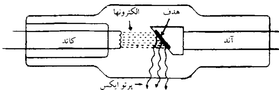
شکل ۲-۴ لوله ساده مولد اشعه ایکس
