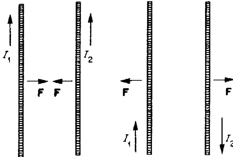
شکل ۶-۱ نیروهای بین سیم های موازی حامل جریان. جریان های همسو نیروی ربایشی و جریان های ناهمسو نیروی رانشی را بوجود می آورد.
