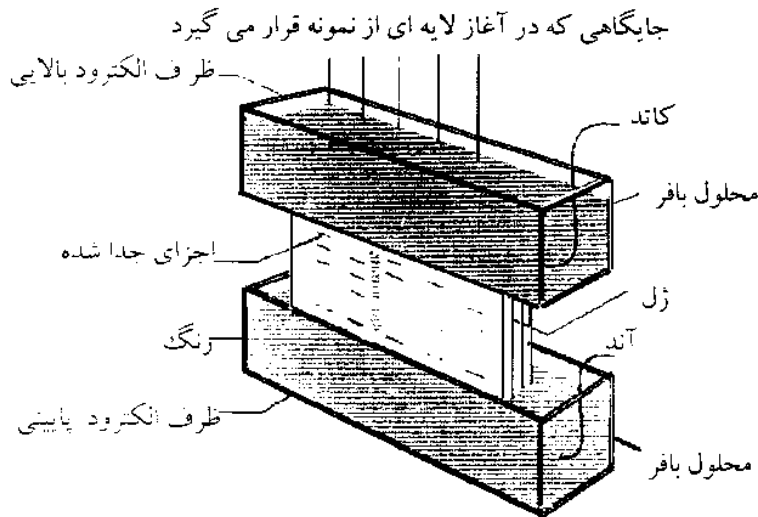
شکل ۱۵-۳ الکتروفورز ژل
