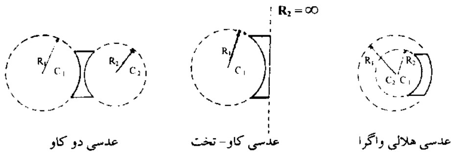
شکل ۸-۲ عدسی های واگرا (مقعر). میان این عدسی ها از کناره های آن نازک تر است.
