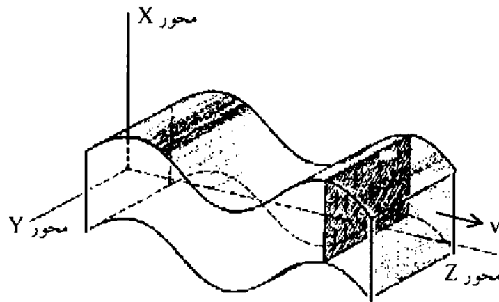
شکل ۹-۱ یک موج تخت سینوسی
