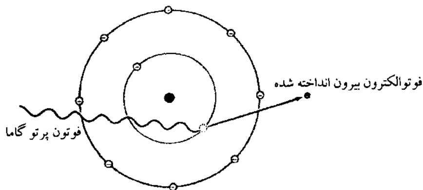
شکل ۷-۴ اثر فوتوالکتریک
