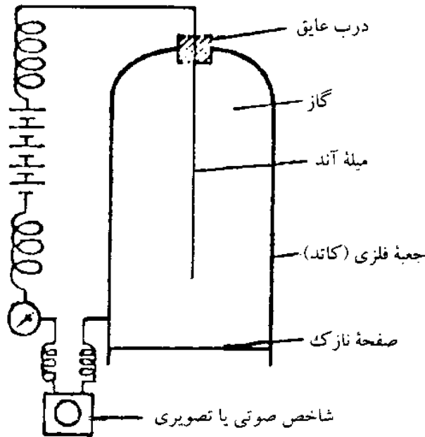
شکل ۷-۸ کنتور گایگر
