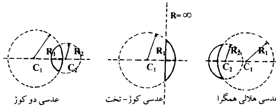
شکل ۸-۱ عدسی های همگرا (محدب). C_2 و C_1 مراکز انحنای وجوه و R_1 و R_2 شعاع های انحنای وجوه عدسی هستند. خط واصل مراکز انحنای وجوه، محور اصلی عدسی و محل تلاقی محور اصلی با عدسی، مرکز اپتیکی نام دارد. میان هر سه عدسی فوق از لبه های آن پهن تر است.
