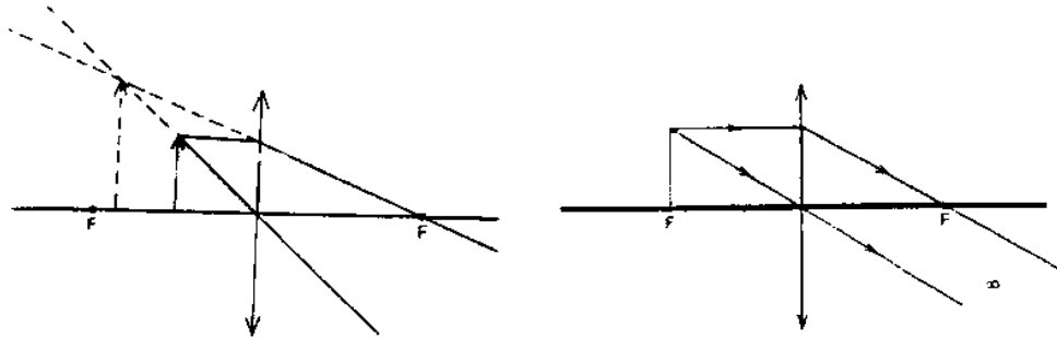
شکل ۸-۵ شیء در کانون، تصویر در بی نهایت.
