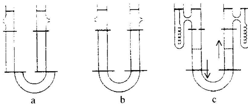
شکل ۱۳-۳ سل U شکل الکتروفورز مرز متحرک
