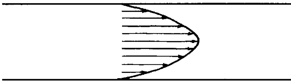
شکل ۳-۶ نمودار سرعت جریان در یک لوله استوانه‌ای
