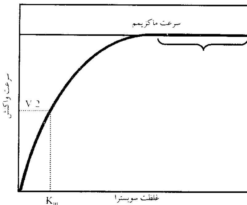
شکل ۳-۲ منحنی اشباع آنزیمی
