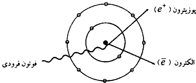
شکل ۶-۷ تولید جفت
