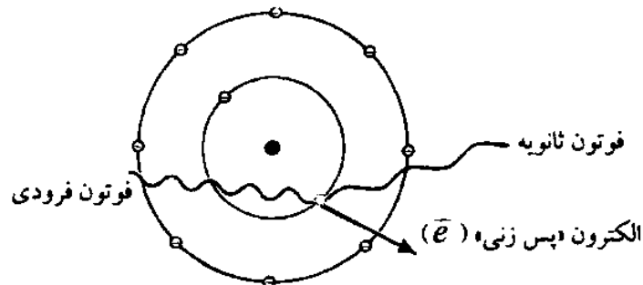
شکل ۵-۷ فرایند کامپتون
