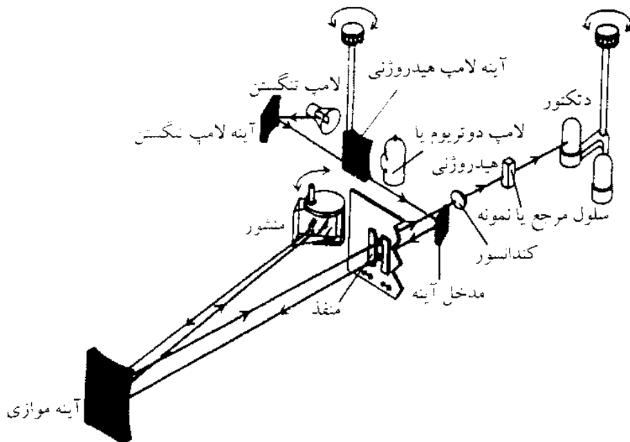
شکل ۱۱-۳ دستگاه اسپکتروفتومتر ناحیه مرئی ساخت کمپانی آمسکو (نک شعاعی).
