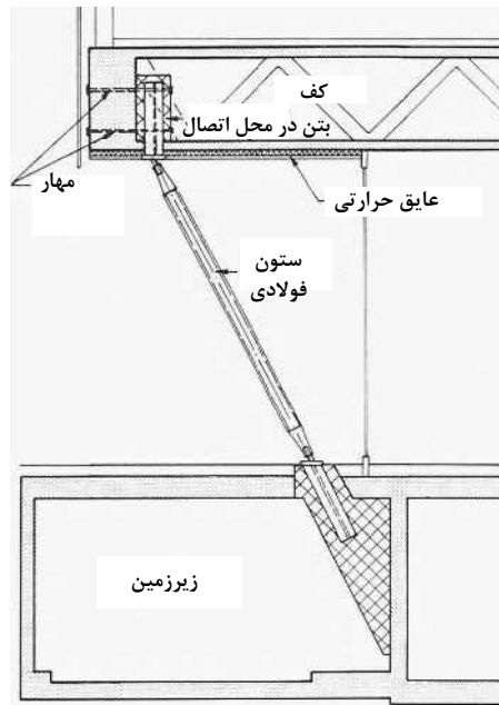
نمایش مقطع خرپای مورب جدید در طبقه همکف (Schefer, Zwicky, Santchi, 1995)
